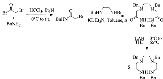
Scheme 5. Synthesis of N,N',N'',N''' -tetrabenzyltriethylenetetraamine ( 5 )
